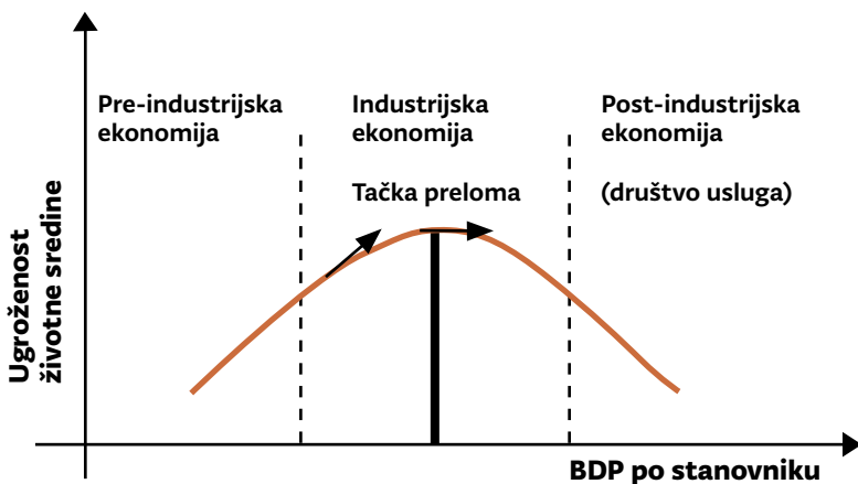
Grafik 8. Ekološka Kuznjecova kriva
